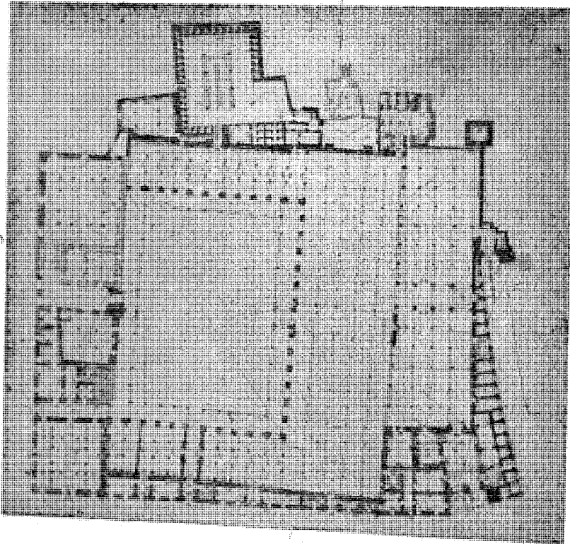
٤ - مستط. أفقي للجامع الأزهر (٩٧٠ - ٩٧٢)
